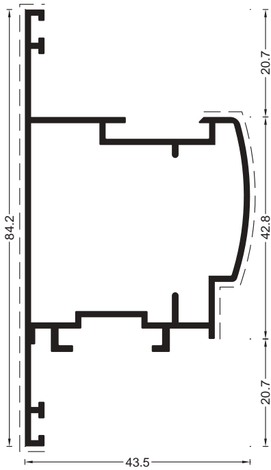
COD 1.31 G=0.92 kg/m P=336 mm Cercevea deschidere exteriora
