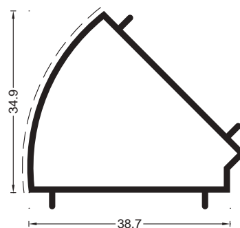
COD 1.33 G=0.45 kg/m P=150 mm Adaptor 45°
