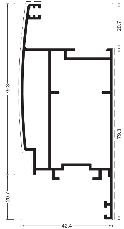
COD 1.35 G=1.20 kg/m P=381 mm Cercevea mare
