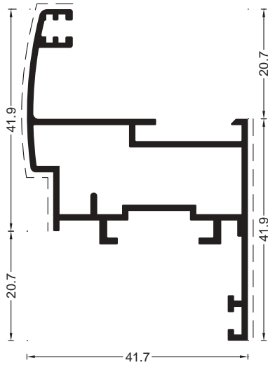
COD 1.26 G=0.73 kg/m P=306 mm Cercevea mica
