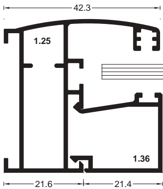
Fereastră cu 1 canat batant / oscilo-batant.
