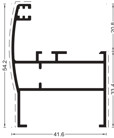
COD 1.39 G=0.73 kg/m P=302 mm Toc mediu
