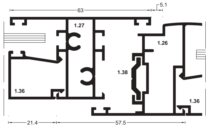
Fereastră cu 2 canate unul fix si unul batant.
