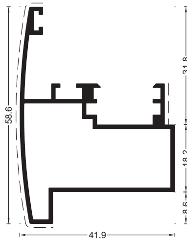
COD 1.34 G=0.74 kg/m P=273 mm Inversor
