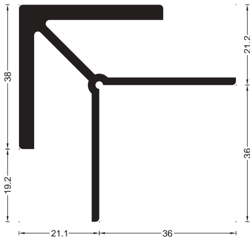
COD 1.40 G=1.45 kg/m P=336 mm Coltar compensare
