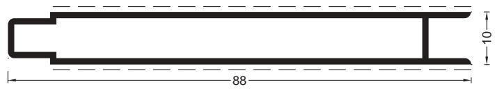
COD 1.21 G=0.31 kg/m P=121 mm Prag
