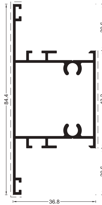
COD 1.30 G=0.96 kg/m P=353 mm Montant - traversa mare
