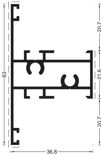
COD 1.27 G=0.79 kg/m P=311 mm Montant - traversa mica
