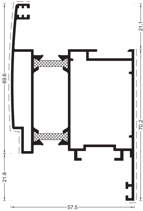
COD 2.21 G=1.48 kg/m P=515 mm Ceravea mare
